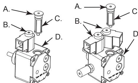
Figure 11 - Pompe du brûleur
