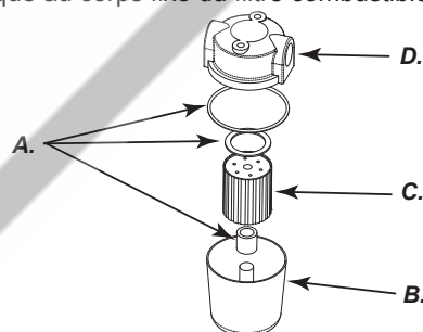
Figure 10 - Filtre en ligne
